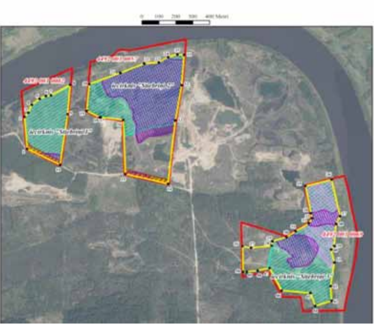
Smilts-grants un smilts atradnes “Elerne” iecirkņa “Stiebrīņi 1”, iecirkņa “Stiebrīņi 2” un iecirkņa “Stiebrīņi 3” izvietojuma plāns
